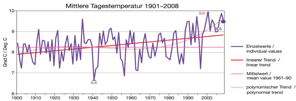
Abb. 3: Jahresmitteltemperatur in Deutschland 1901-2008. Es gab zwar schon immer Schwankungen, es lässt sich jedoch erkennen, dass die letzten 15 Jahre überdurchschnittlich warm waren. Vor allem aber ist der jüngste Anstieg seit etwa 1970 stärker als jemals vorher in der Datenreihe / nach Deutscher Wetterdienst, 2009).
