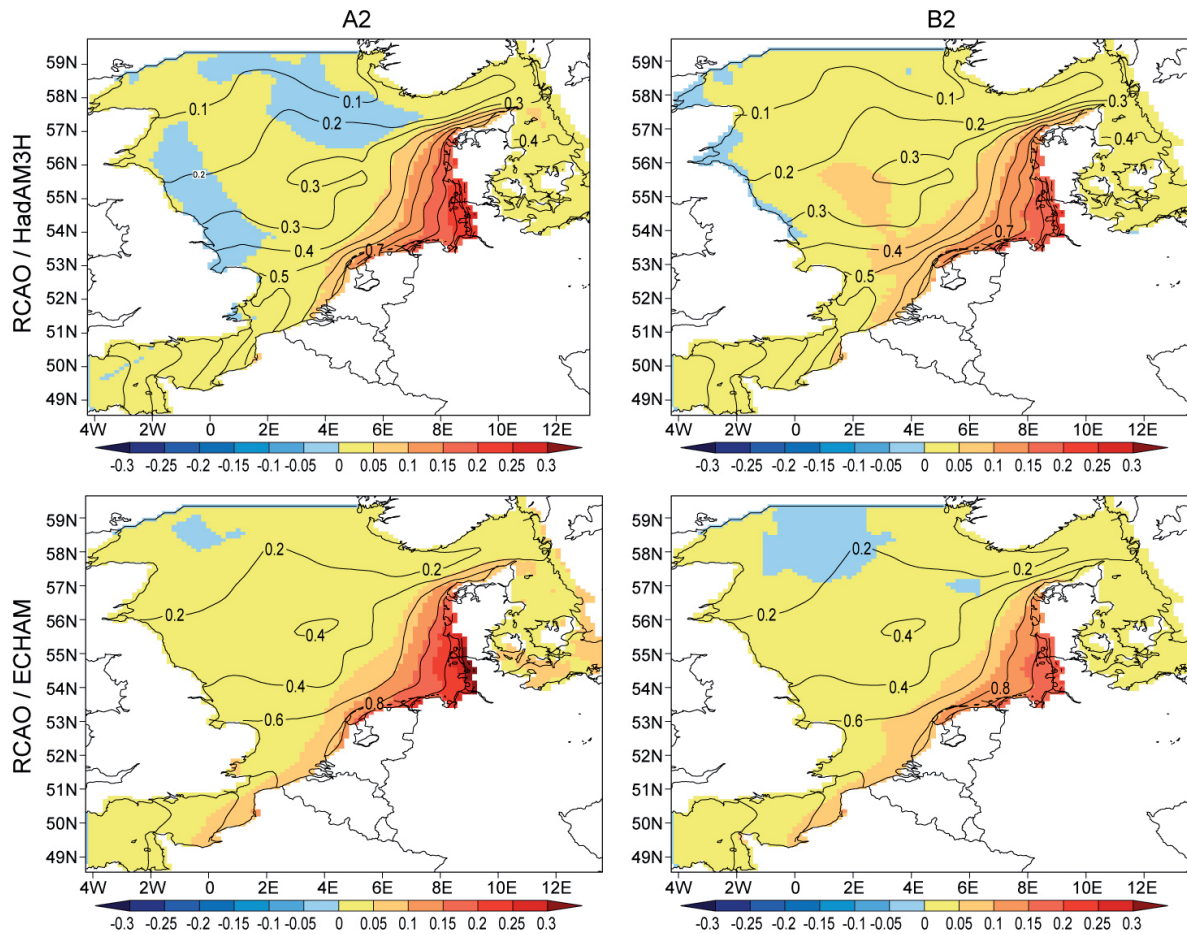
Abb. 10: Erwarteter Effekt veränderter Sturmtätigkeit über der Nordsee auf die Windstauhöhen. Atmosphärischer Antrieb: zwei unterschiedliche Emissionsszenarien. A2 in der linken Spalte und B2 in der rechten Spalte. Die Zeilen zeigen die jeweiligen regionalen Klimarechnungen mit Antrieben von zwei verschiedenen globalen Klimamodellen. Regionalisiert wurde mit dem regionalen Atmosphärenmodell des SMHI (Schwedisches Institut für Hydrologie und Meteorologie). Das Sturmflutmodell der GKSS berechnet aus der regionalen Atmosphäre schließlich die Wasserstände. Dargestellt ist die Änderung der Erwartung hoher Wasserstände (99,5 Perzentil) (Farbskala) im Vergleich zur heutigen Sturmflutklimate Situation (Isolinien). Einheit: Meter (aus Woth und von Storch 2008).
