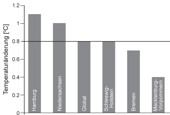
Abb. 4: Änderungen der Temperatur in Norddeutschland berechnet aus Temperaturmessungen des letzten Jahrhunderts. Es wurden die Messwerte aller verfügbaren Messstationen gemittelt (nach I. Meinke 2008, pers. Komm.).
