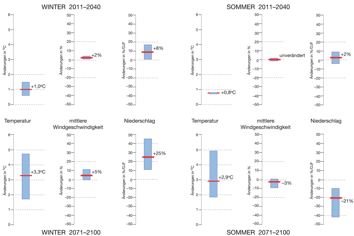
Abb. 8: Regionale Klimaszenarien für die Nordseeküste. Gezeigt werden mögliche Änderungen der Temperatur für die Emissionsszenarien A2 und B2 (Mittel, Minimum, Maximum), der maximalen Windgeschwindigkeiten und der monatlichen Summe der Niederschläge in Norddeutschland (Mittelwerte des Gebietes Schleswig-Holstein, Hamburg, Niedersachsen). Oben: Zeithorizont 2040; Unten Zeithorizont 2100. Rechts: Sommermonate (Juni, Juli, August); Links: Wintermonate (Dezember, Januar, Februar). (Norddeutscher Klimaatlas, www.norddeutscher-klimaatlas.de ).
