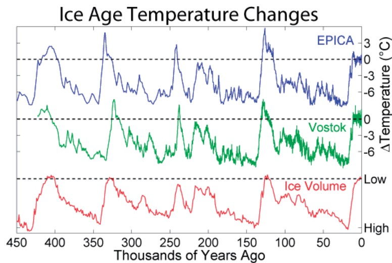
Abb. 2: Die beiden oberen Kurven der Abbildung zeigen die Änderung der geschätzten Temperatur an zwei Stellen in der Antarktis während der Glaziale/Interglaziale des Quartärs und als Vergleich in der unteren Kurve das geschätzte Anwachsen und Abschmelzen der globalen Eismassen. An den Kurven lässt sich eindeutig die hohe Korrelation von Temperaturänderungen in der Antarktis und dem Volumen der globalen Eismassen und damit dem Meeresspiegel ablesen (Abbildung erstellt von Robert A. Rohde / www.globalwarmingart.com ).
